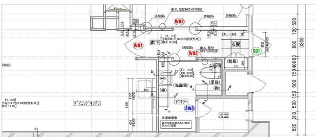
平面図
